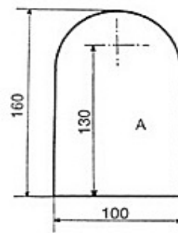
Schéma 4 : PIÈCES D'ARTICULATION ET RENFORTS (Tôle d'acier de 3 mm)
